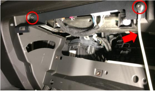
Installation de la gâche et du câble de retenue
